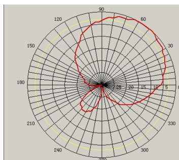
E-Plane
